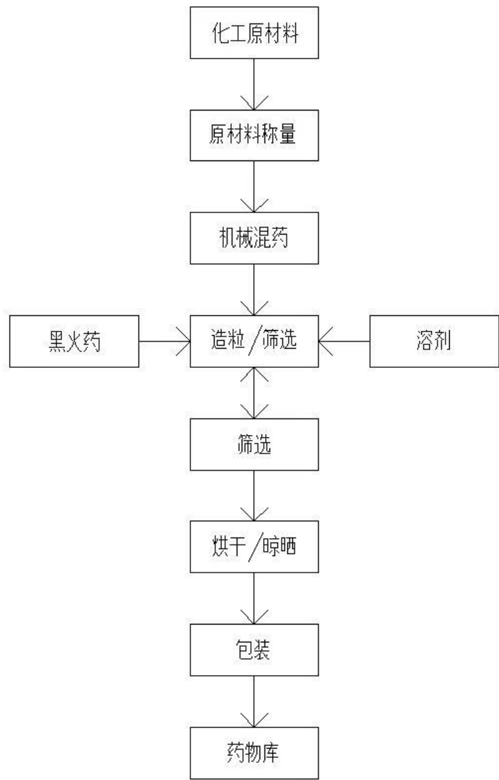
烟火药类（亮珠）生产工艺流程图
