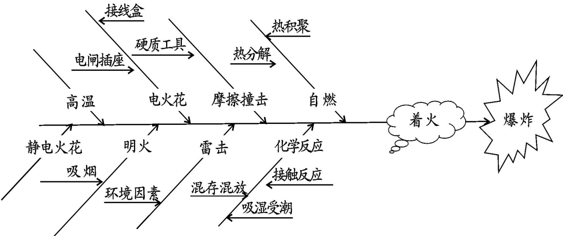
图 3-1 烟花爆竹引爆的因果分析图
