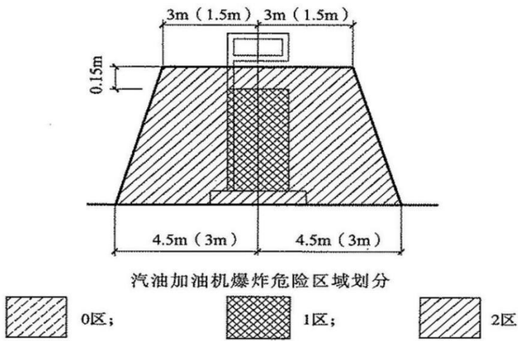
图 3.6-1 汽油加油机爆炸危险区域划分图
